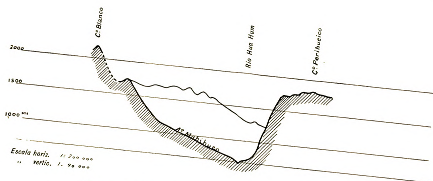
FIG. 4.— DIAGRAMA DEL CORTE DEL RÍO HUAHUM.
