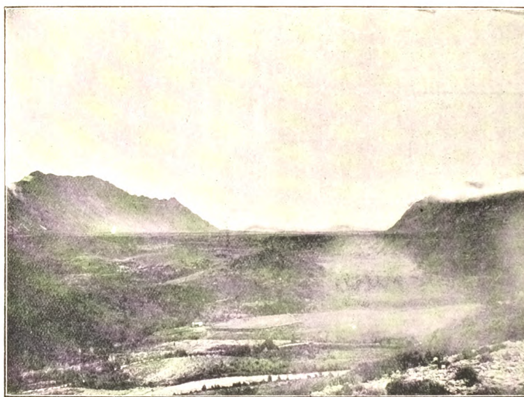
FIG. 6.—DIVORCIO CONTINENTAL ENTRE LOS RIOS QUENQUENTREU Y MAITEN.
