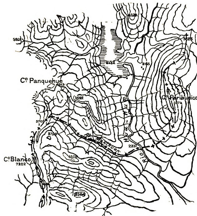
FIG. 2.—CORTE DEL RÍO HUAHUM POR LA LÍNEA FRONTERIZA ARGENTINA.
